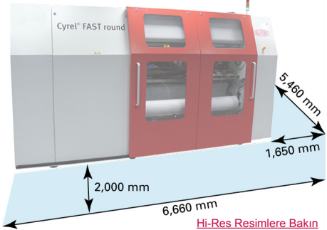
Makine Yerleşim Planı
